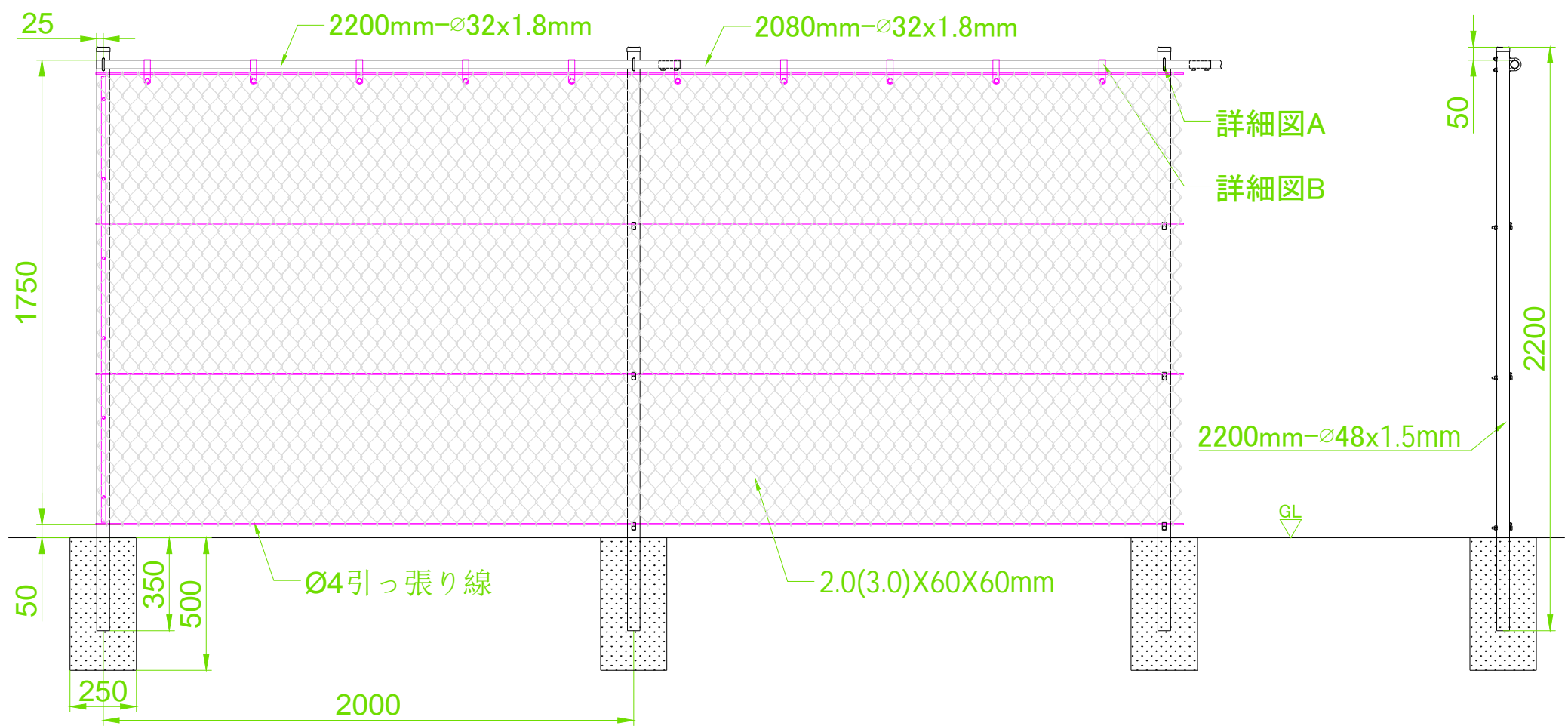
正立面図
