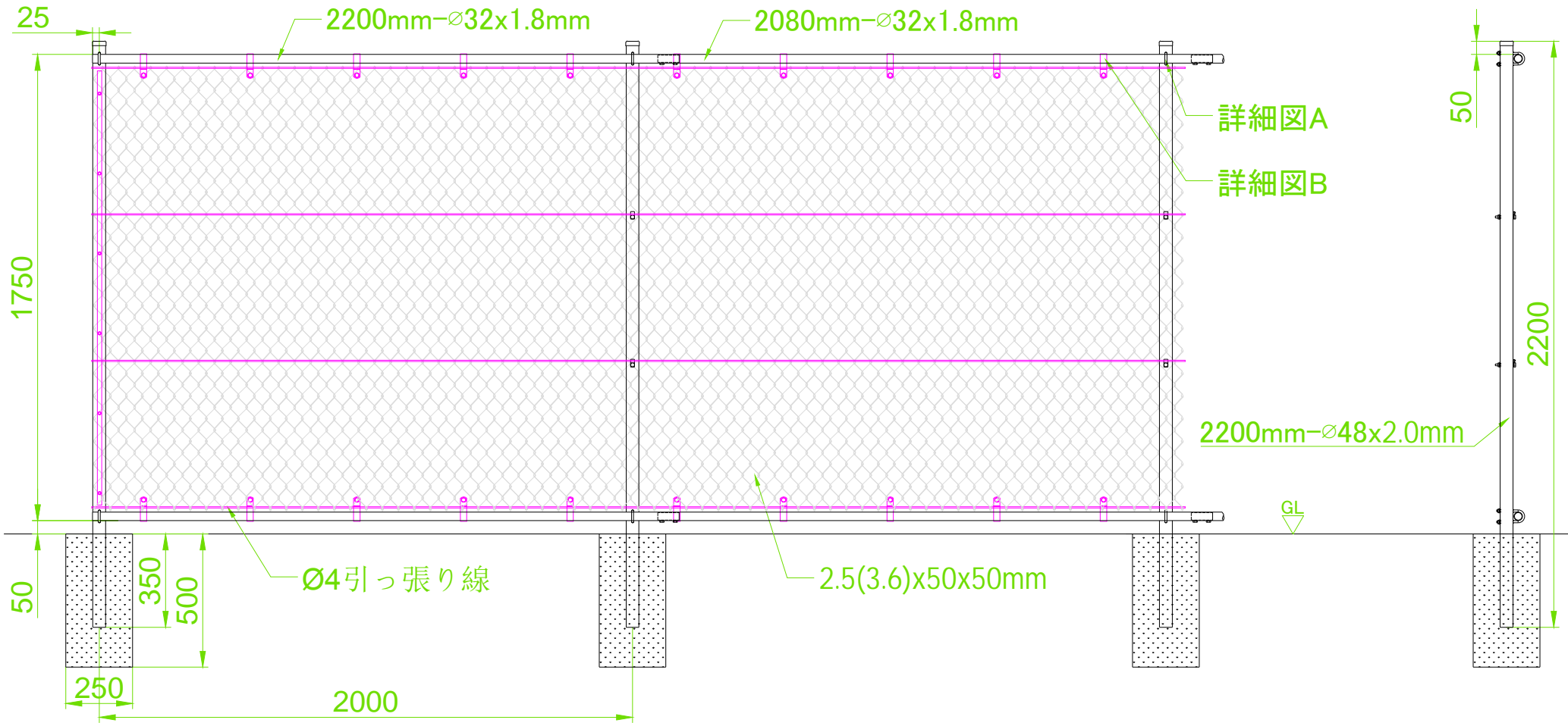
正立面図
