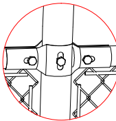
詳細図A
